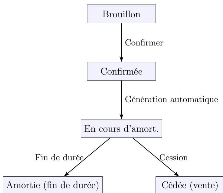
FIGURE 1 – Diagramme d'états – Cycle de vie d'une immobilisation
