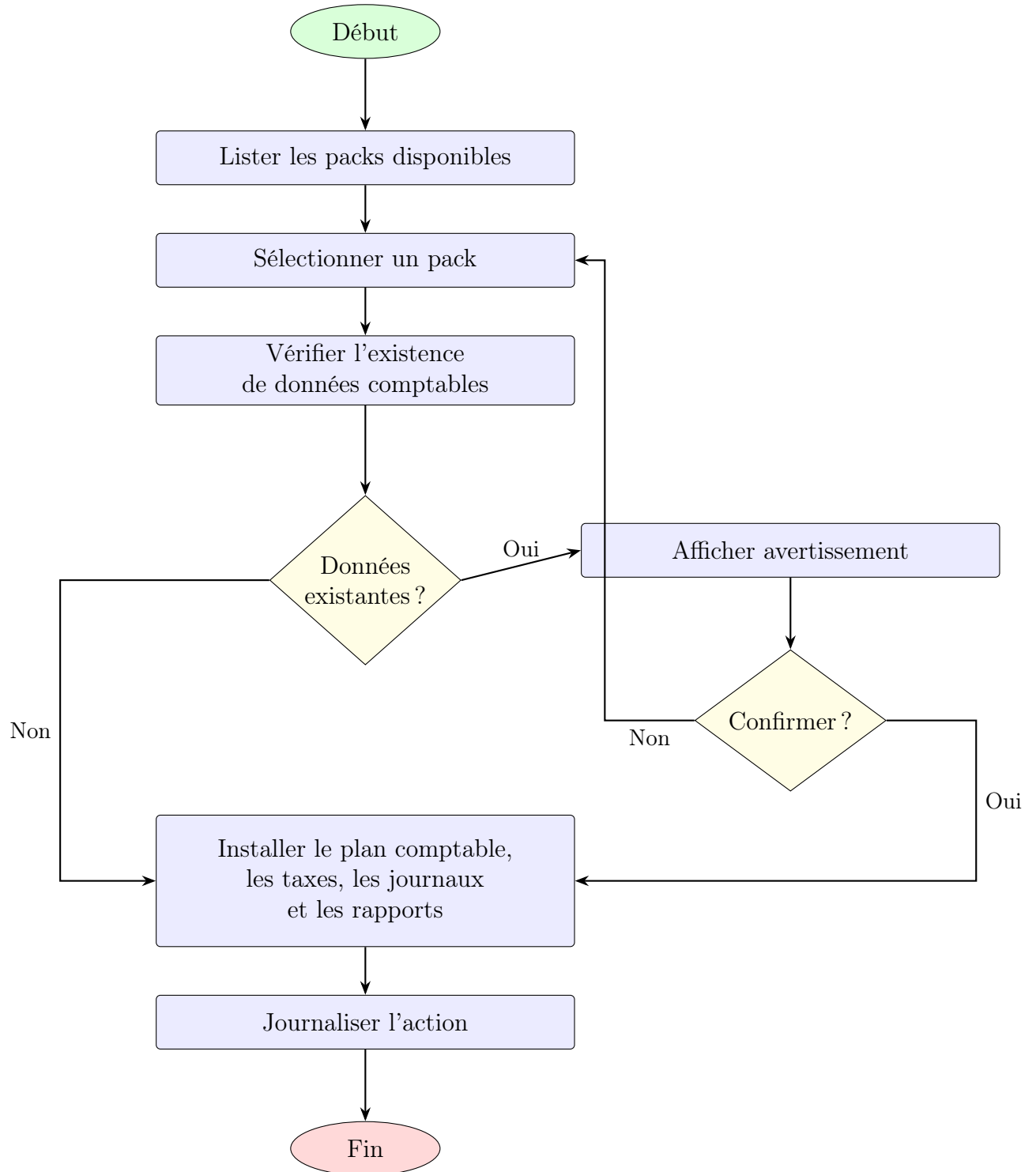
FIGURE 2 – Diagramme d'activité – Processus d'installation d'un pack de localisation
